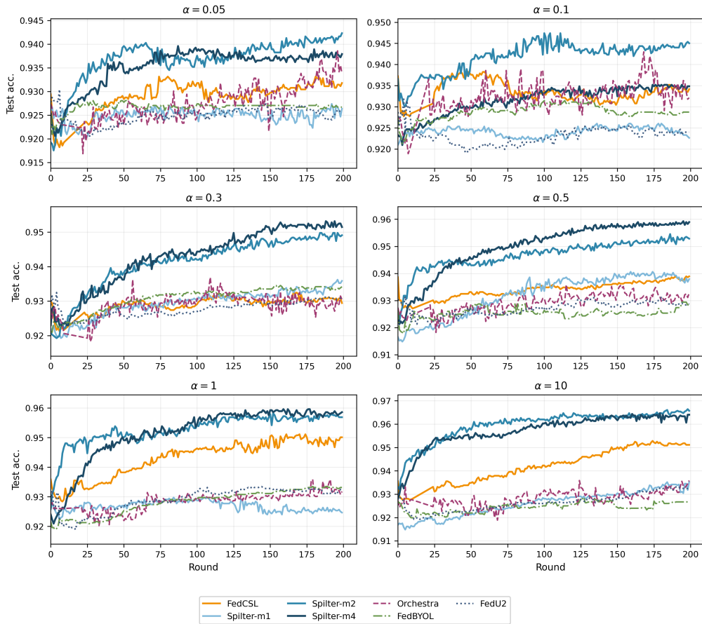
Figure 4: HAR 数据集上不同 Dirichlet 参数 \alpha 下各联邦学习方法的测试准确率随通信轮次变化曲线（3×2 子图：自上而下、自左而右对应 \alpha = 0.05, 0.1, 0.3, 0.5, 1.0, 10.0 ；Spilter 按 local\_top\_m \in \{1, 2, 4\} 画为三条曲线；各子图纵轴按该 \alpha 下曲线范围自适应放大）。数据来自 data/HAR/alpha_* 真实训练日志。
